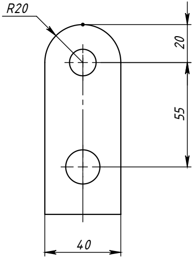
Поз.3 (Серьга) 1:2
